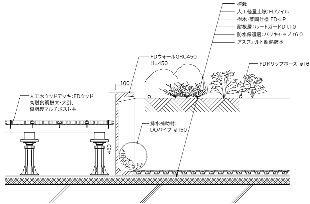
5. 樹木・菜園仕様 FD-LP
