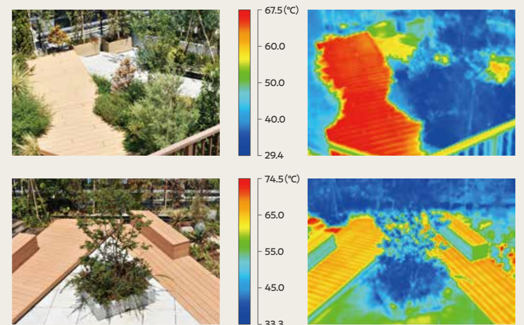
田島ルーフィング 小台研修センター 屋上緑化 10ページ掲載の屋上緑化展示場を、赤外線サーモグラフィで計測してみました。 緑化面積 164.21m 2 計測日 2023年7月26日 上:ハーブエリア付近 下:多目的広場付近
