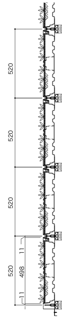
A断面(山部)
