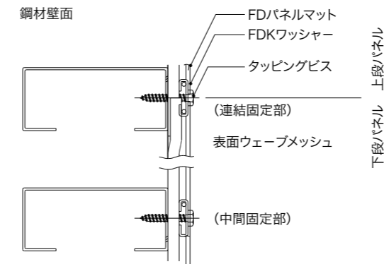
固定部(鋼材壁面)拡大断面図
