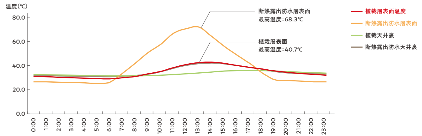
三菱電機(株)稲沢製作所 第15工場屋上緑化 緑化面積 5161.2m 2 緑化仕様 FD-LE(土厚80mm) 計測日 2008年8月12日
