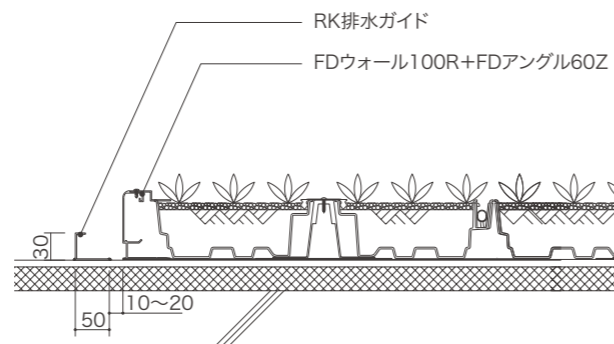
FDウォール100R+RK排水ガイドによる排水イメージ
